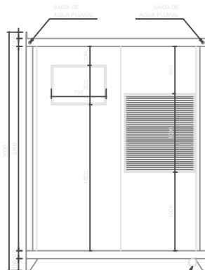
ELEVAÇÃO 03 ESCALA 1:25
