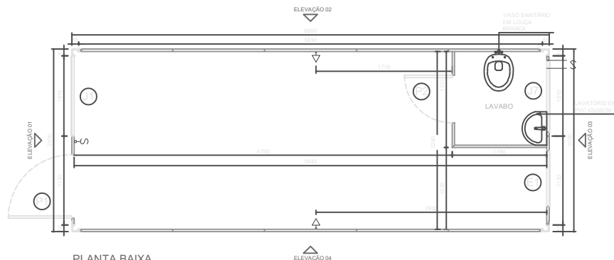
PLANTA BAIXA ESCALA 1:25
