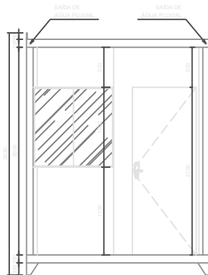
ELEVAÇÃO 01 ESCALA 1:25
